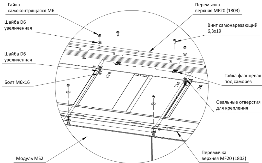
Крепление модуля к перемычкам верхним, вид сзади
